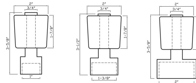
D2009 A Fits 1" Rod
