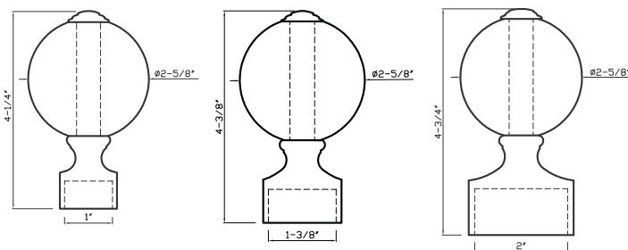
D2004 A Fits 1" Rod
