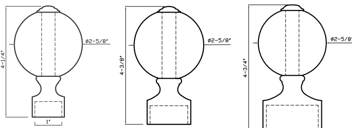
D2021 A Fits 1" Rod
